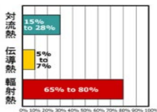
壁(横)からの熱移動
